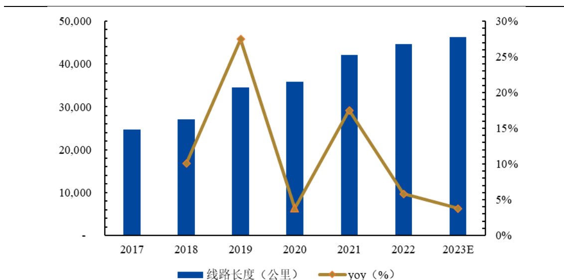
图表：中国特高压工程累计线路长度及预测
