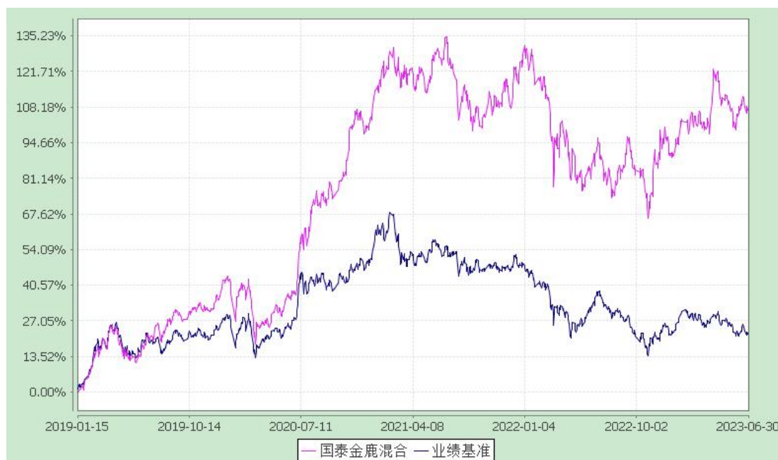
国泰金鹿混合型证券投资基金 累计净值增长率与业绩比较基准收益率历史走势对比图 (2019 年 1 月 15 日至 2023 年 6 月 30 日)
