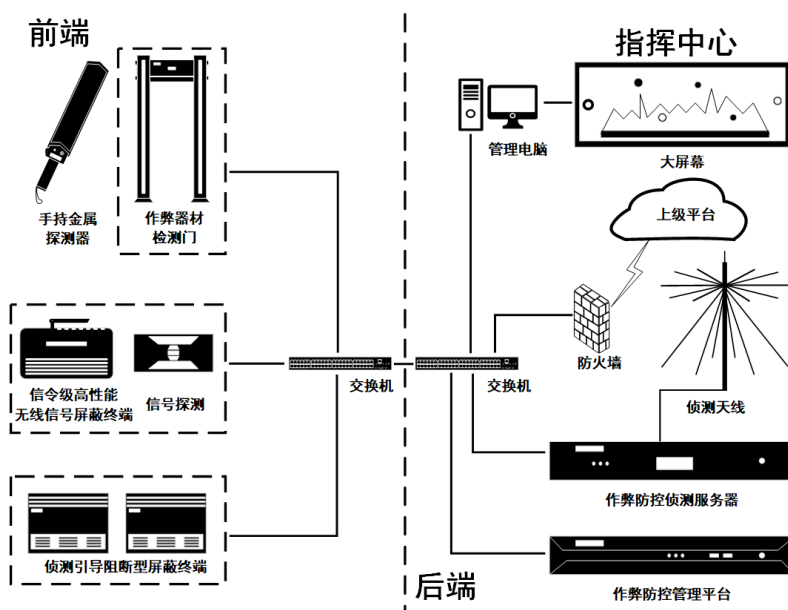
作弊防控系统示意图
