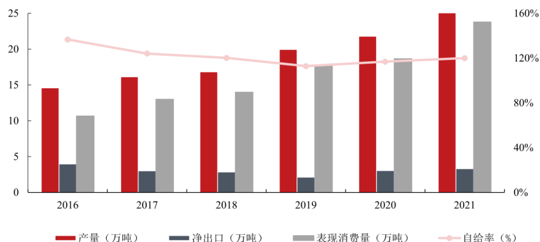
2016 年以来我国主要含氟高分子材料产品产量
