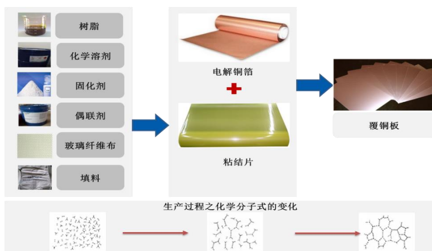
覆铜板和粘结片的关系
