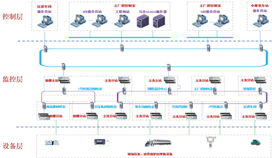
图 14：综合自动化系统网络
