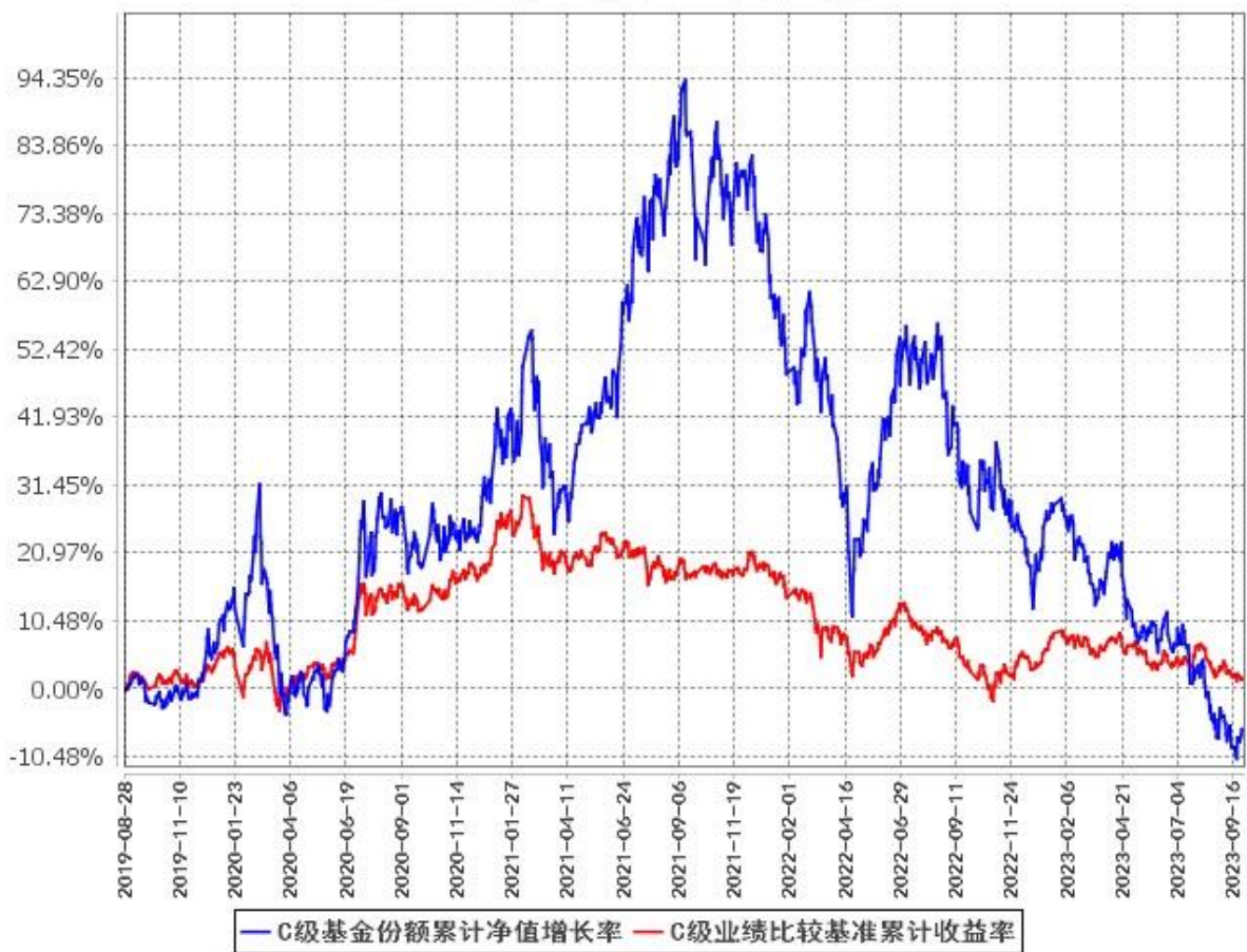
C级基金份额累计净值增长率与同期业绩比较基准收益率的历史走势对比图 (2019年8月28日至2023年9月30日)
