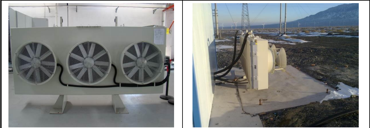
空冷器外观
