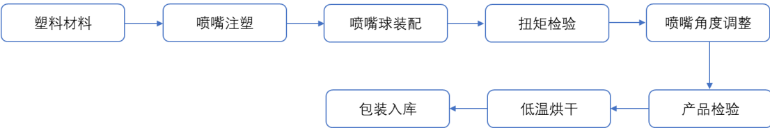
④ 加液管生产流程图
