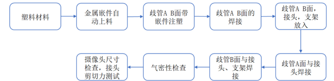
(4) 冷却歧管产品生产流程图
