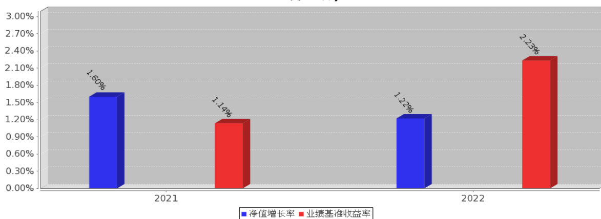
嘉实方舟6个月滚动持有债券发起A基金每年净值增长率与同期业绩比较基准收益率的对比图(2022年12月31日)
