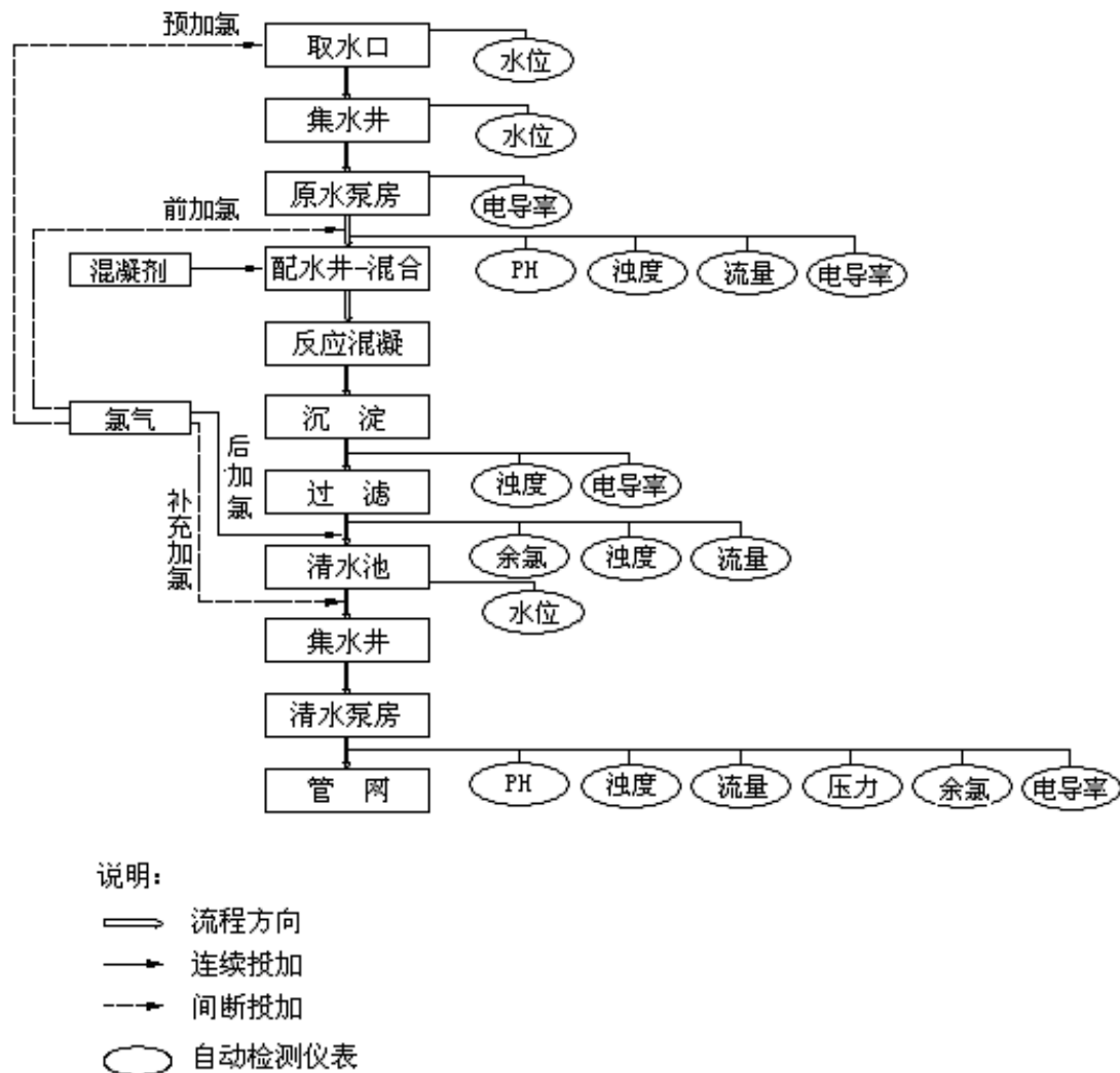
图：供水业务工艺流程
