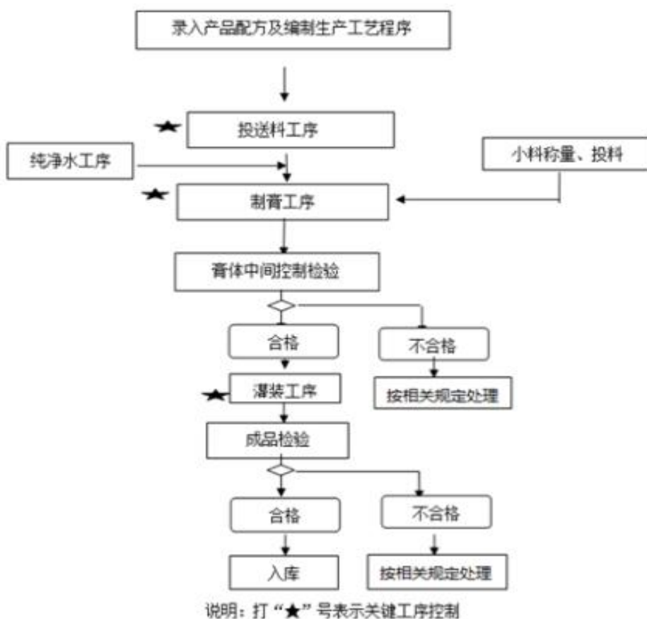
牙膏生产工艺流程图：
