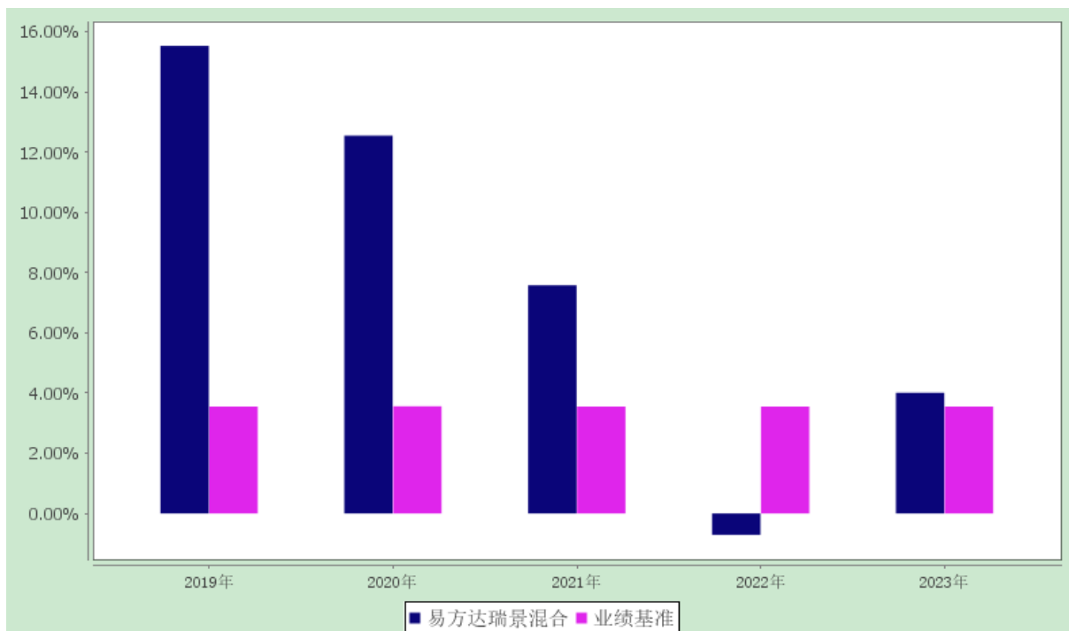
易方达瑞景灵活配置混合型证券投资基金 过去五年基金净值增长率与业绩比较基准历年收益率对比图
