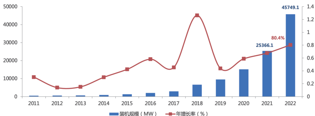
全球新型储能市场累计装机规模（2000-2022）
