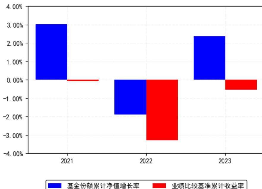
南方宝恒混合A每年净值增长率与同期业绩比较基准收益率的对比图（2023年12月31日）
