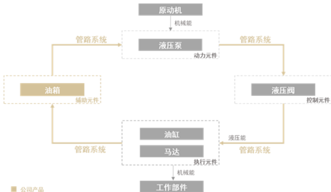
液压系统工作原理图
