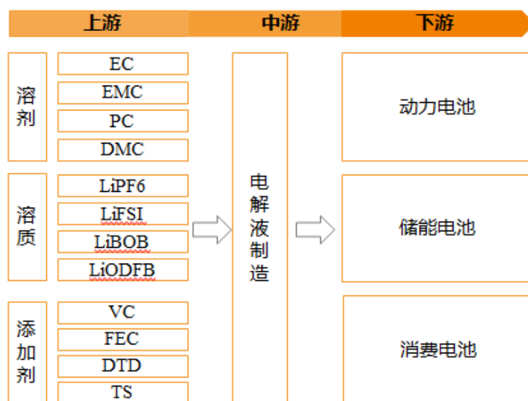
锂电池电解液产业链结构示意图
