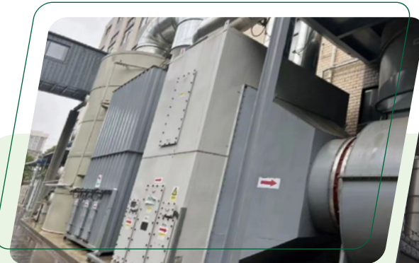
正在工作的 VOCs 废气处理设备
