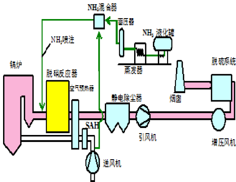
选择性催化还原脱氮 SCR 技术工艺流程
