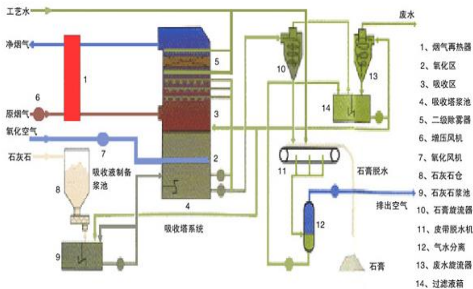
旋汇耦合湿法脱硫工艺流程图
