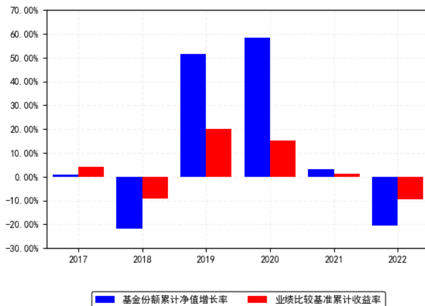
南方平衡配置混合每年净值增长率与同期业绩比较基准收益率的对比图（2022年12月31日）
