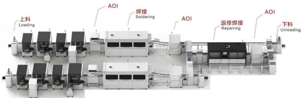
图：零缺陷焊接检测制造系统示意图
