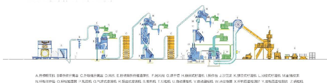
图 1：公司机采棉加工全程机械化、智能化、信息化工艺流程
