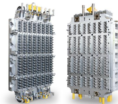
图 2：176 腔瓶坯模具
