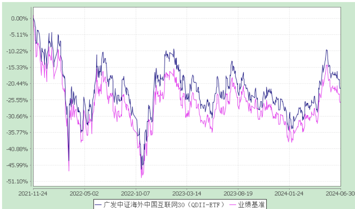
广发中证海外中国互联网 30 交易型开放式指数证券投资基金 (QDII) 份额累计净值增长率与业绩比较基准收益率历史走势对比图 (2021 年 11 月 24 日至 2024 年 6 月 30 日)
