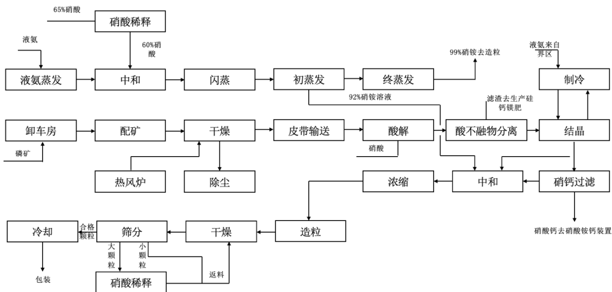
(3) 硝酸铵钙工艺流程
