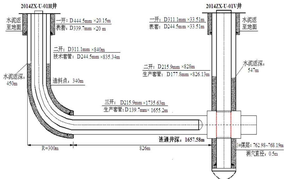
图 U 型井示意图
