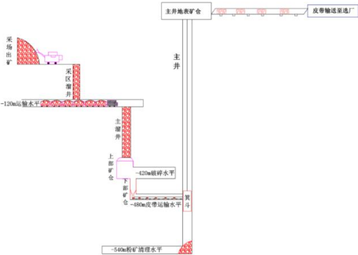
地下采矿生产工艺流程示意图
