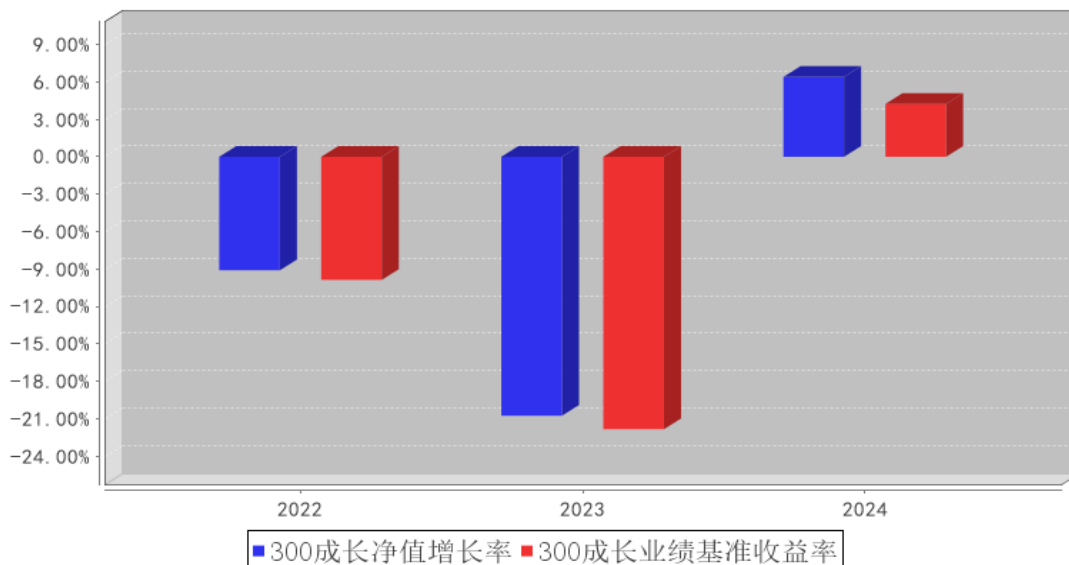
300成长基金每年净值增长率与同期业绩比较基准收益率的对比图
