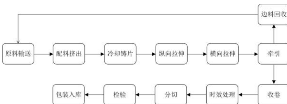
图：功能基膜材料主要工艺流程
