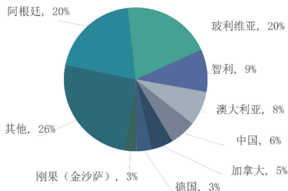
2024年全球锂资源量情况
