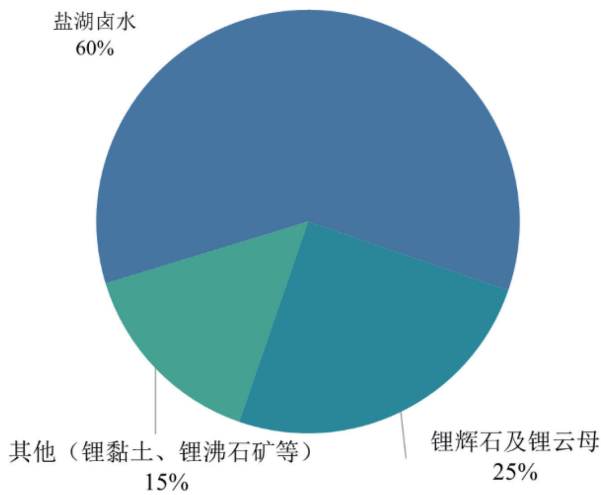
2024年全球锂资源类型分布
