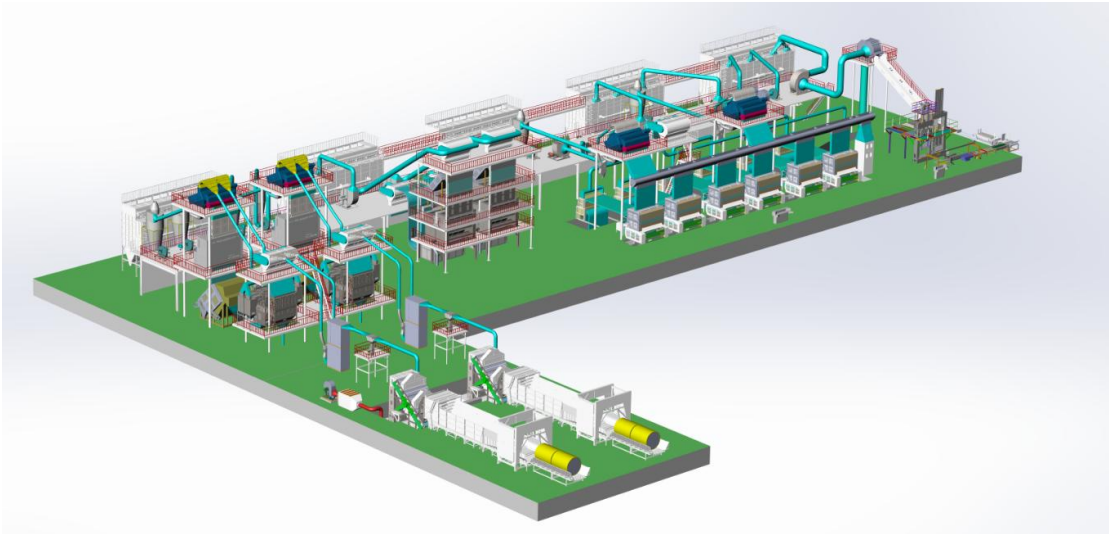
图 1：公司机采棉加工全程机械化、智能化、信息化工艺流程
