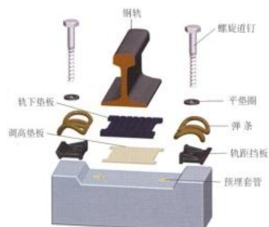
弹条Ⅴ型扣件组装零件图
