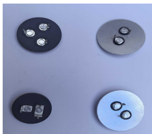
端子（牛角）电容器盖板
