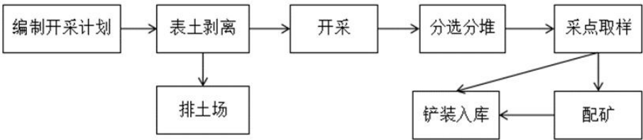
采矿的工艺流程图
