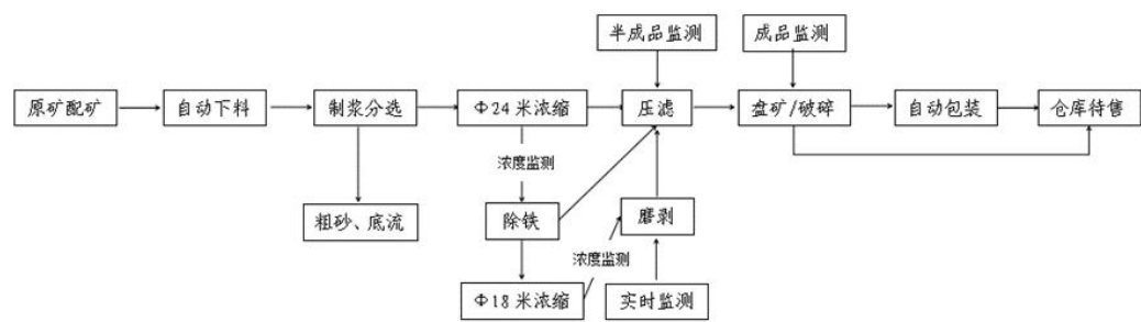
选矿的工艺流程图
