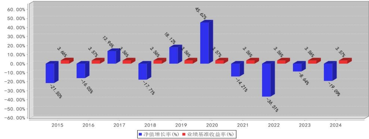
太平灵活配置基金每年净值增长率与同期业绩比较基准收益率的对比图（2024年12月31日）
