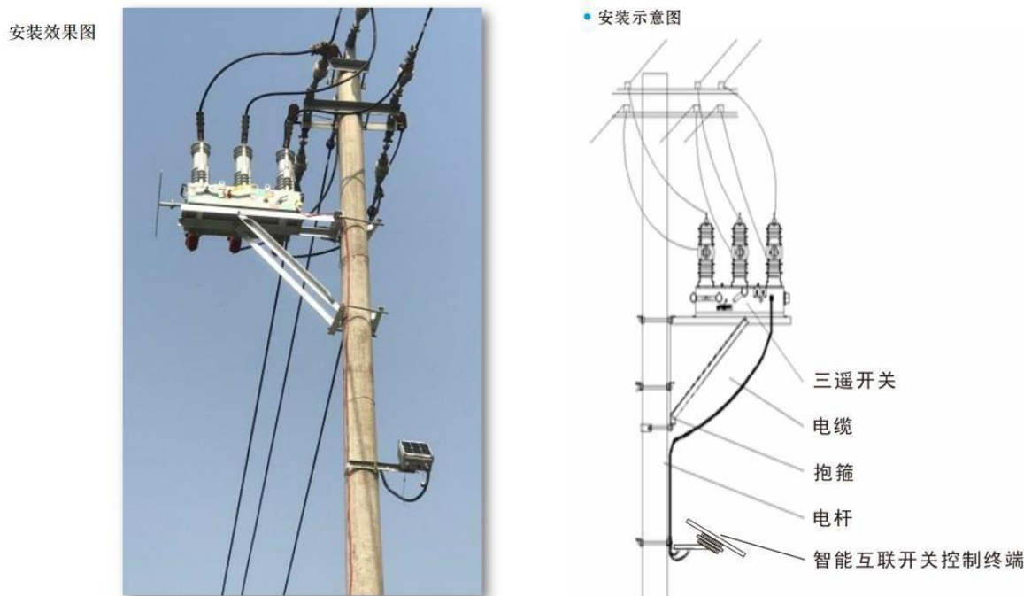
图 2 智能柱上开关安装效果及示意图
