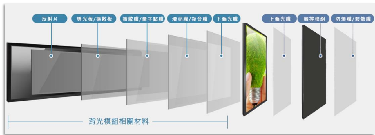
背光模组结构图
