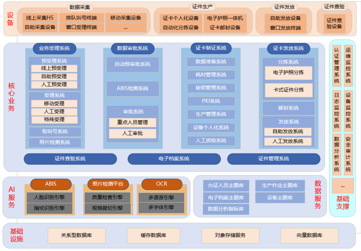
安全证件签发平台-系统架构图
