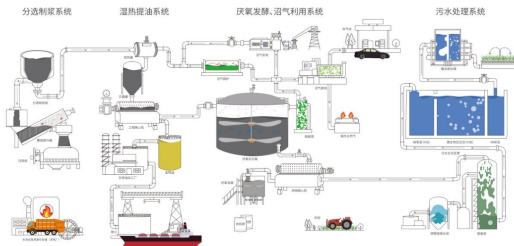
图 3：公司餐厨垃圾处置工艺流程图
