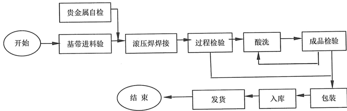
⑧电子束焊生产流程图
