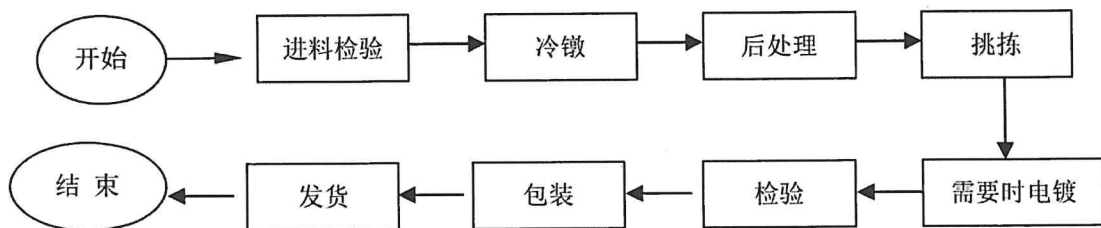
② 铆钉生产流程图
