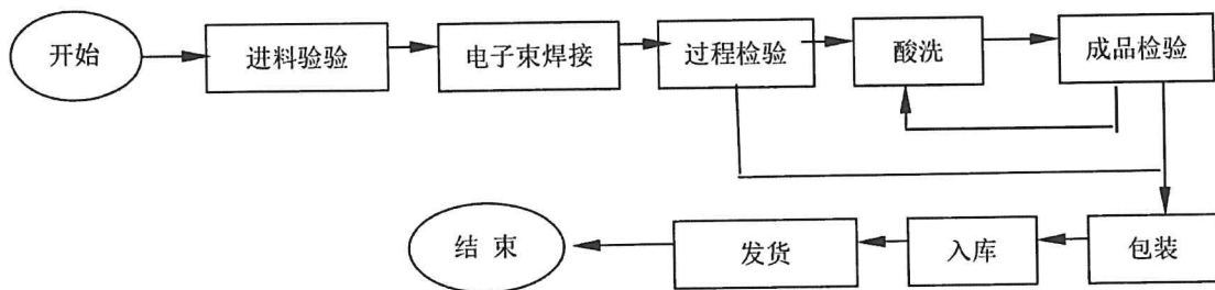
⑨异性丝生产流程图
