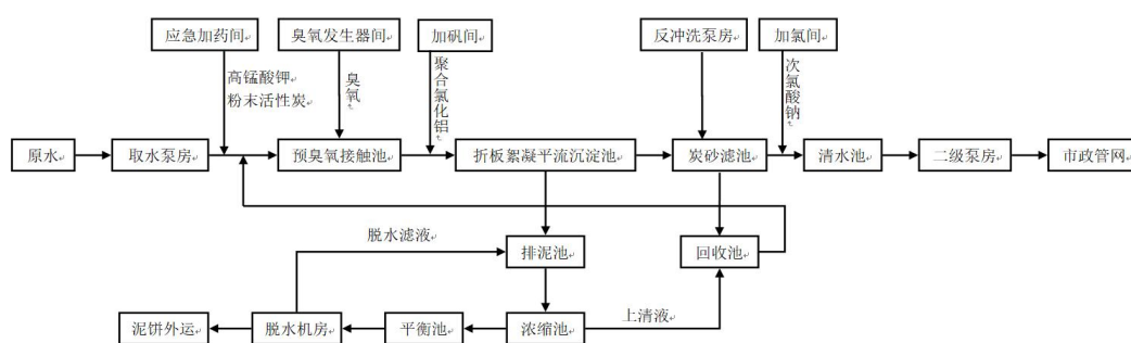
肖山水厂工艺流程图
