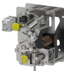
环网柜断路器单元操作机构
