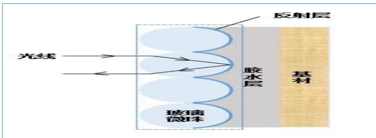
玻璃微珠型反光原理
