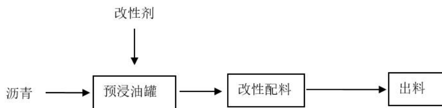
②预浸油配制工艺流程图
