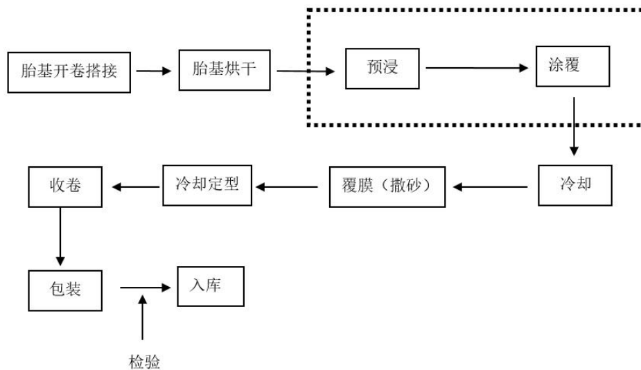
③成型生产工艺流程图
