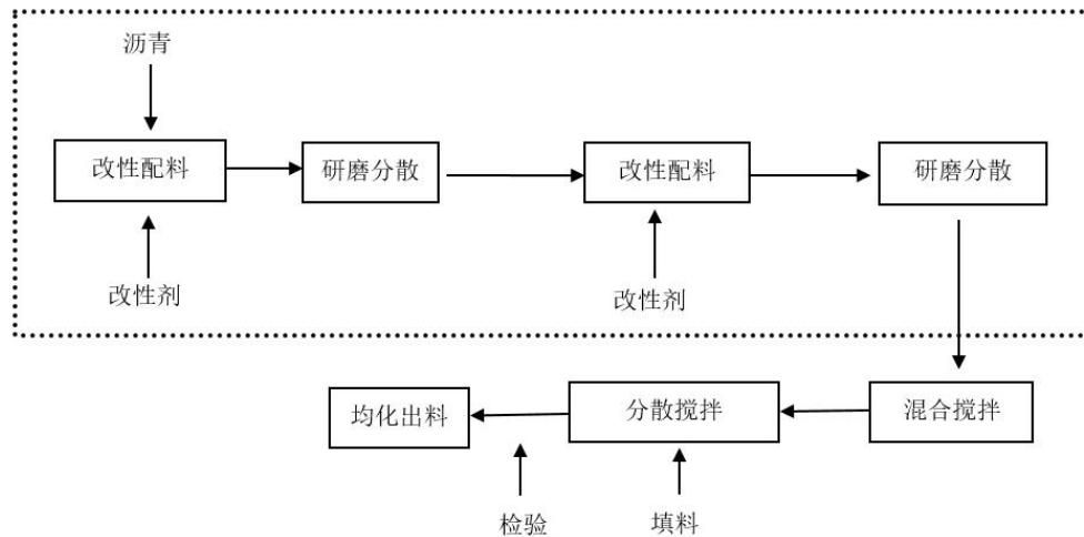
②预浸油配制工艺流程图
