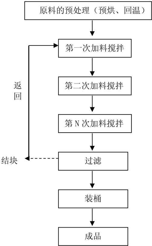
4、光伏封装胶膜产品的工艺流程
