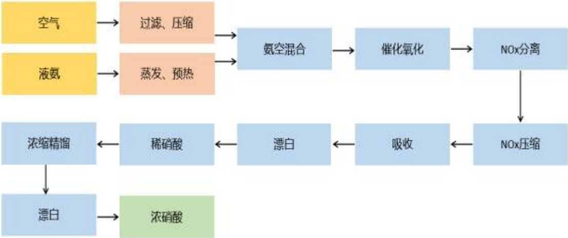
液体硝酸铵的生产工艺流程图
