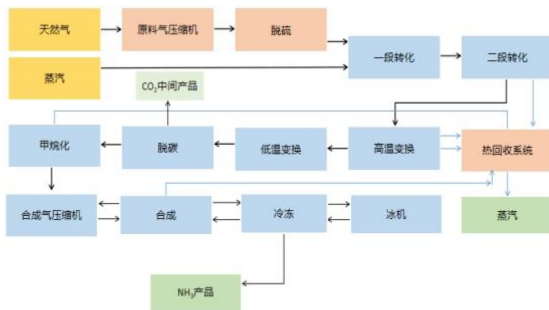
液氨的生产工艺流程图
