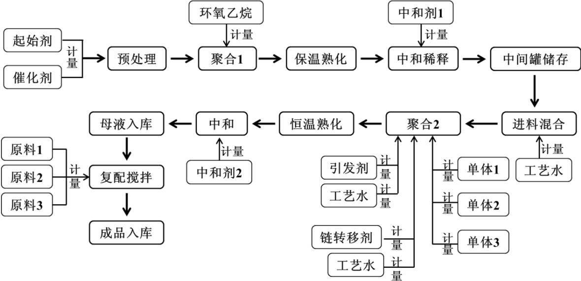
聚羧酸高性能减水剂生产工艺流程图：
