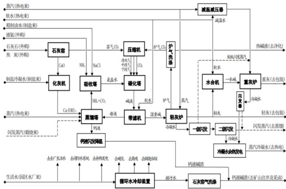
纯碱生产工艺流程图
