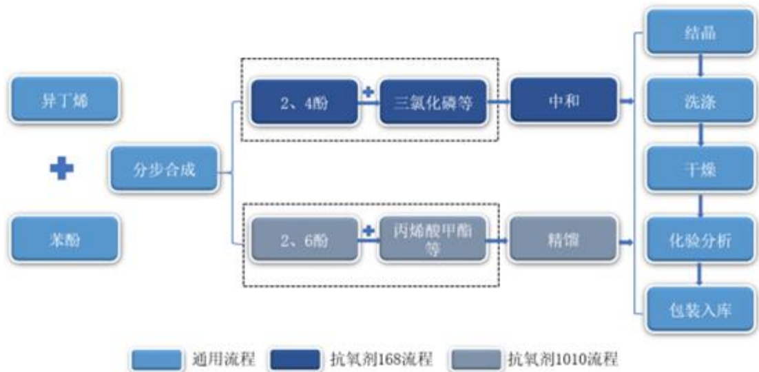
(3) 复合助剂产品生产工艺：
