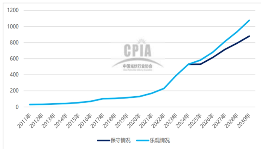
2011-2024 年全球光伏年度新增装机规模以及 2025-2030 年新增规模预测 (单位: GW)
